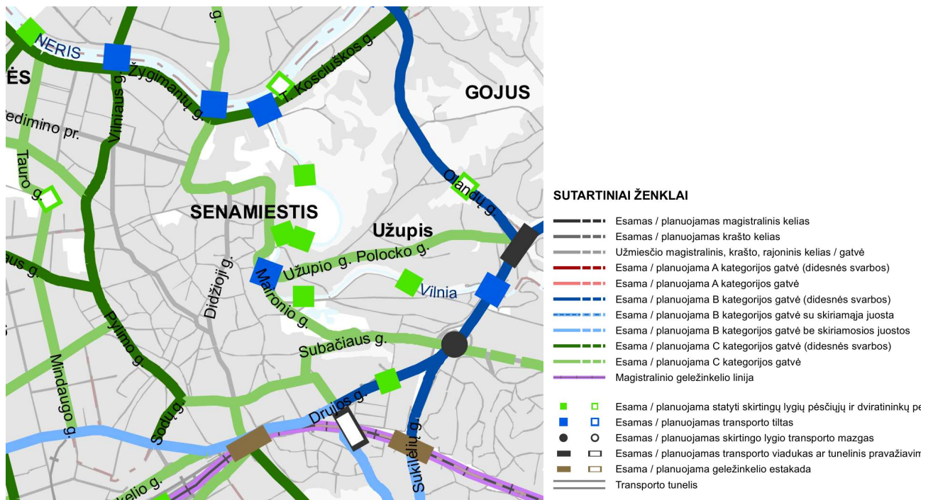
3. pav. Ištrauka iš Vilniaus miesto bendrojo plano brėžinio „Susisiekimas. Gatvių kategorijos“
